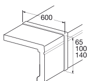
Profils d'assemblage pour tablettes de fenêtre
