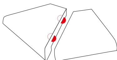
Assemblage en onglet avec lamellos **
