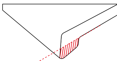
Fraiser le bord avant à fleur ****
