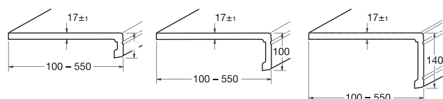
Caches du système
