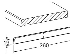
Caches de finition
