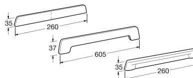
exclusiv Capuchons de finition
