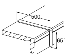
Profilés d'assemblage pour tablettes de fenêtre
