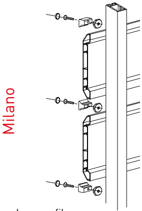
Langprofil
