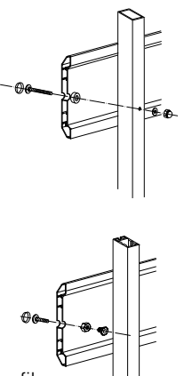
Langprofil
