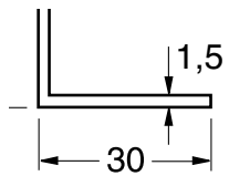
Abdeckwinkel 30/20
