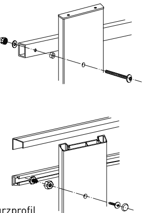
Kurzprofil
