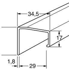
Kantenprofil B
